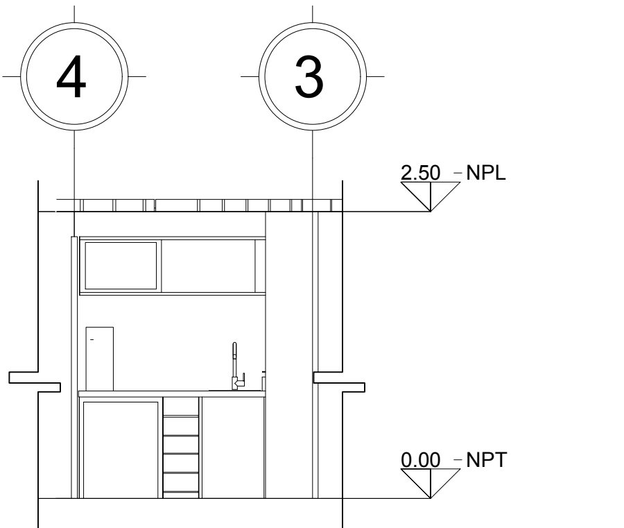
CORTE G-G' - COCINA
