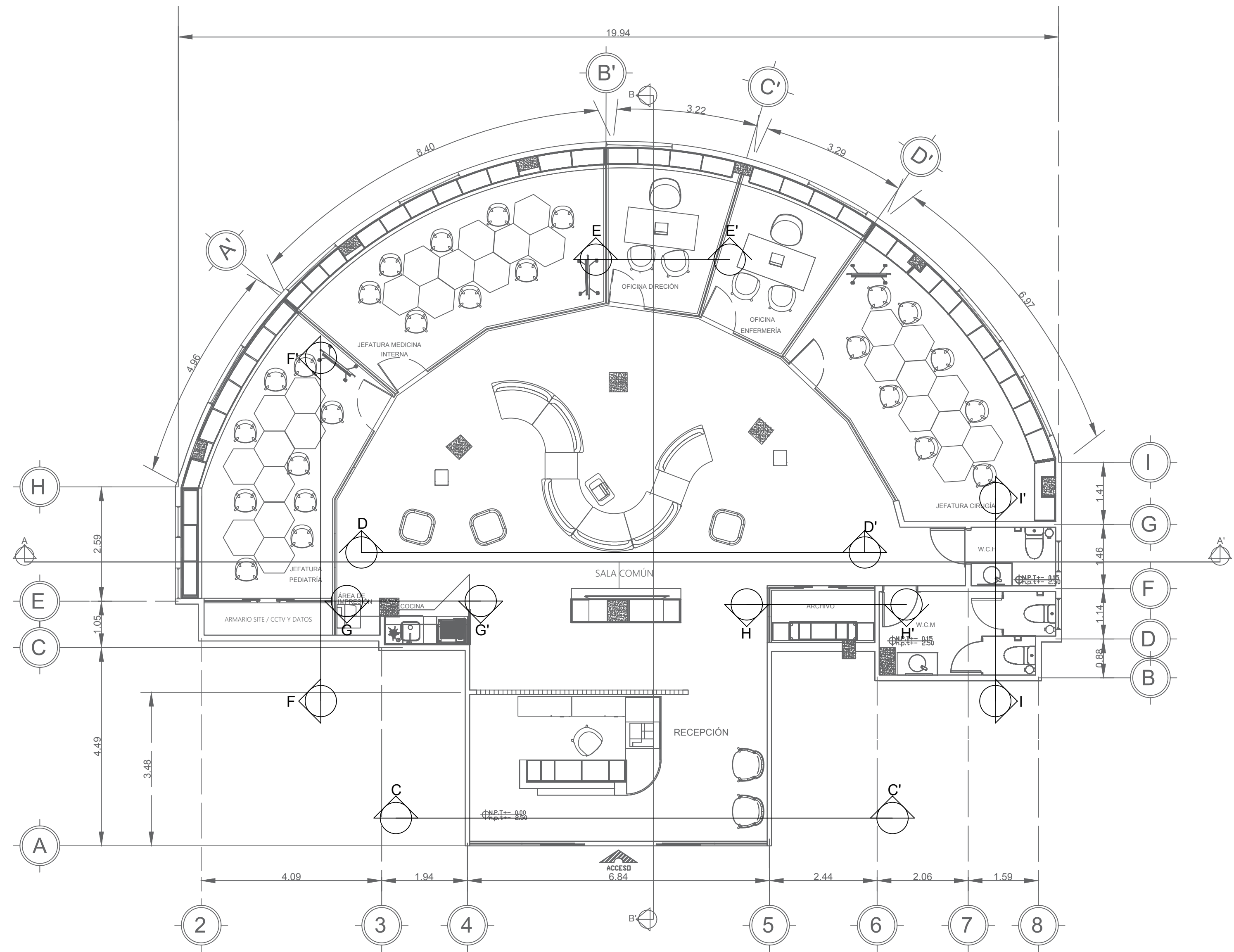
PLANTA ARQ. CON CORTES
