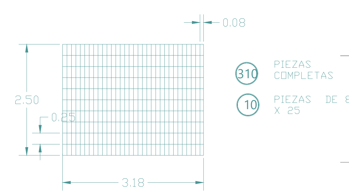
DETALLE 2 DE COLOCACIÓN DE AZULEJOS EN MURO SANITARIO MUJERES
