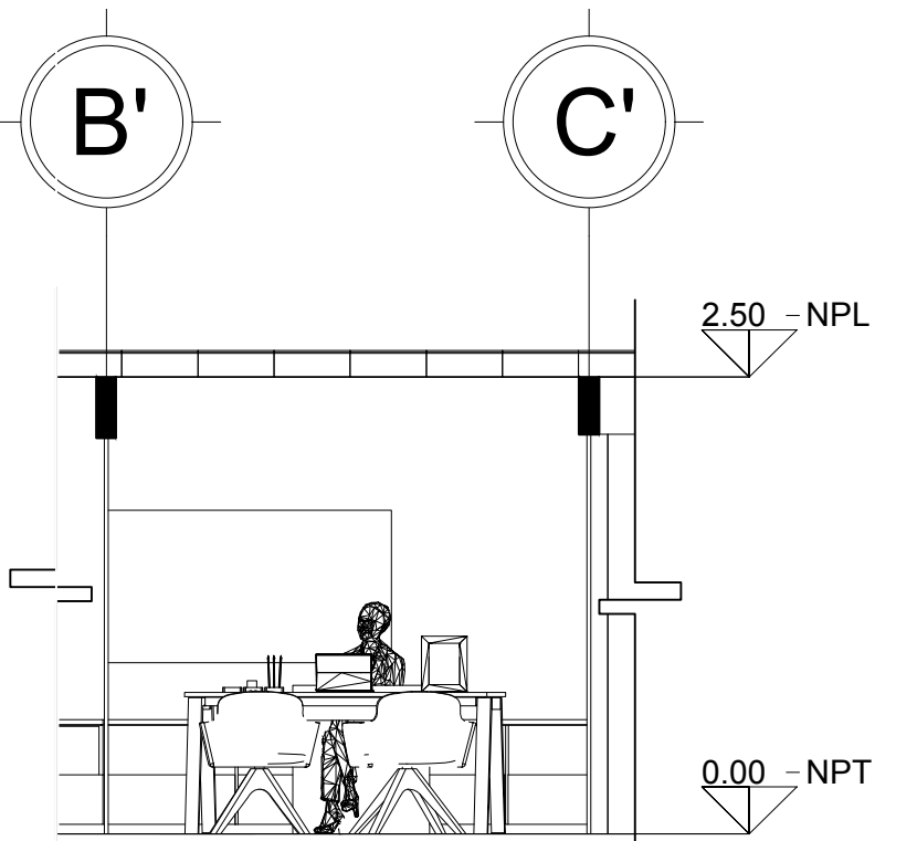
CORTE E-E' - OFICINA
