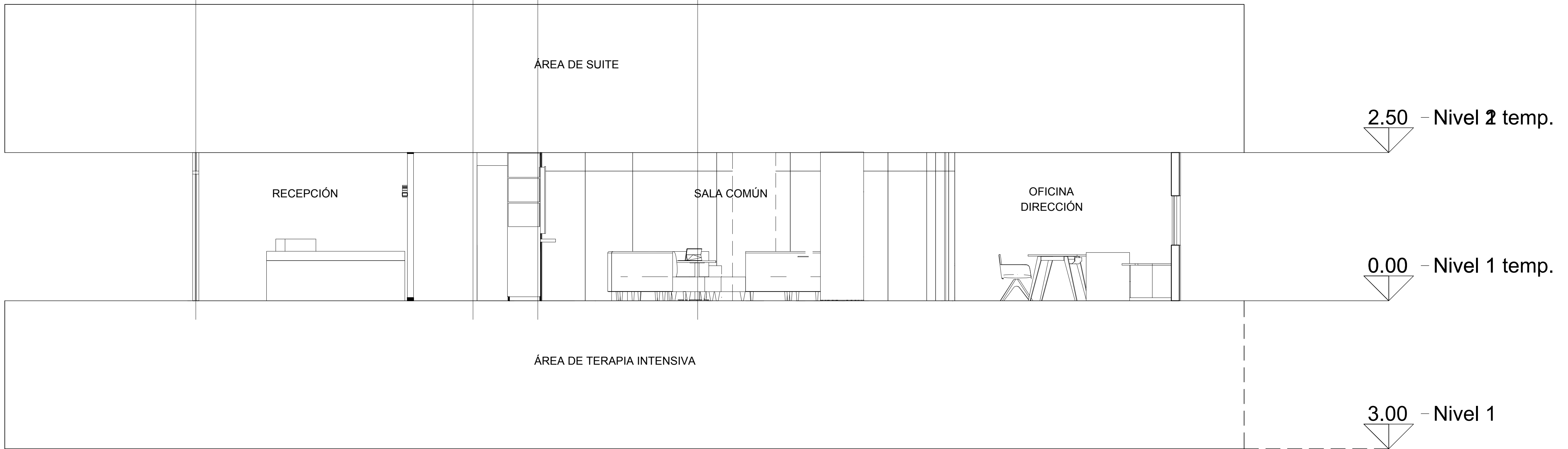
CORTE B-B' TRANSVERSAL
