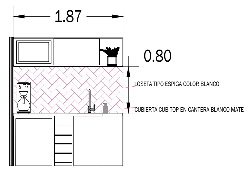
ÁREA DE COCINA VISTA FRONTAL
