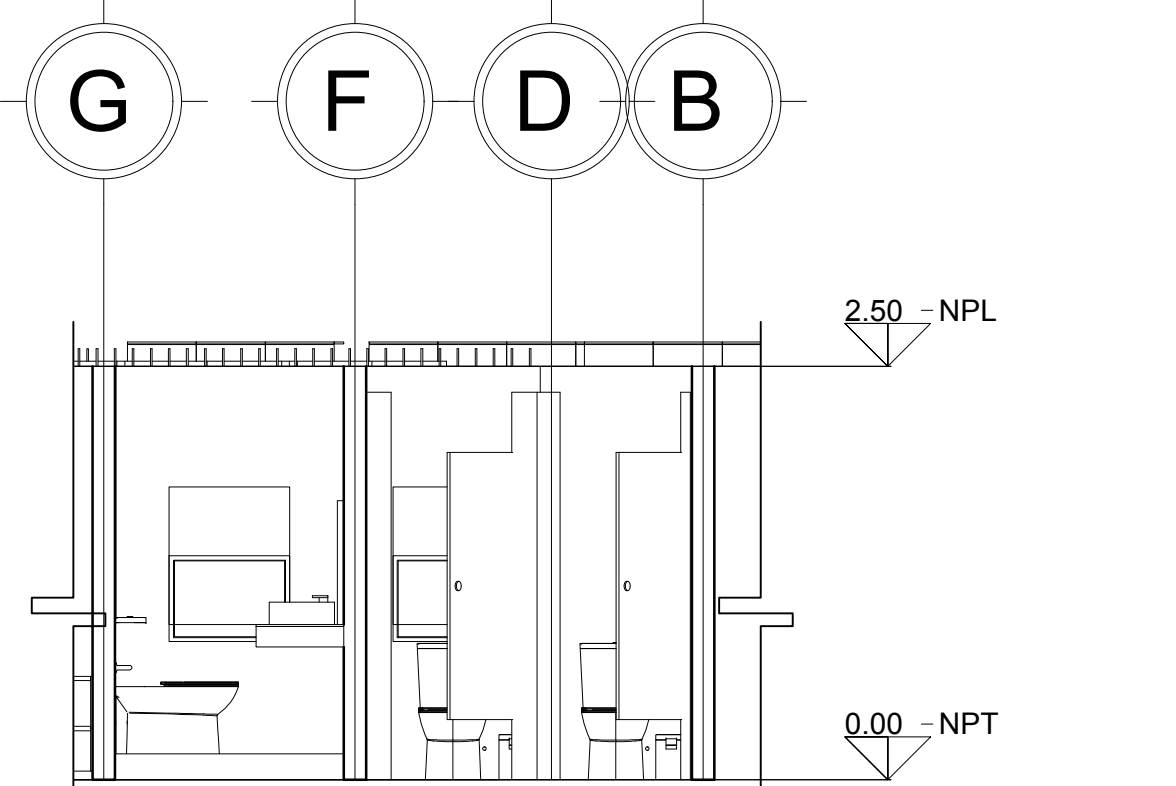
CORTE I-I' - BAÑOS
