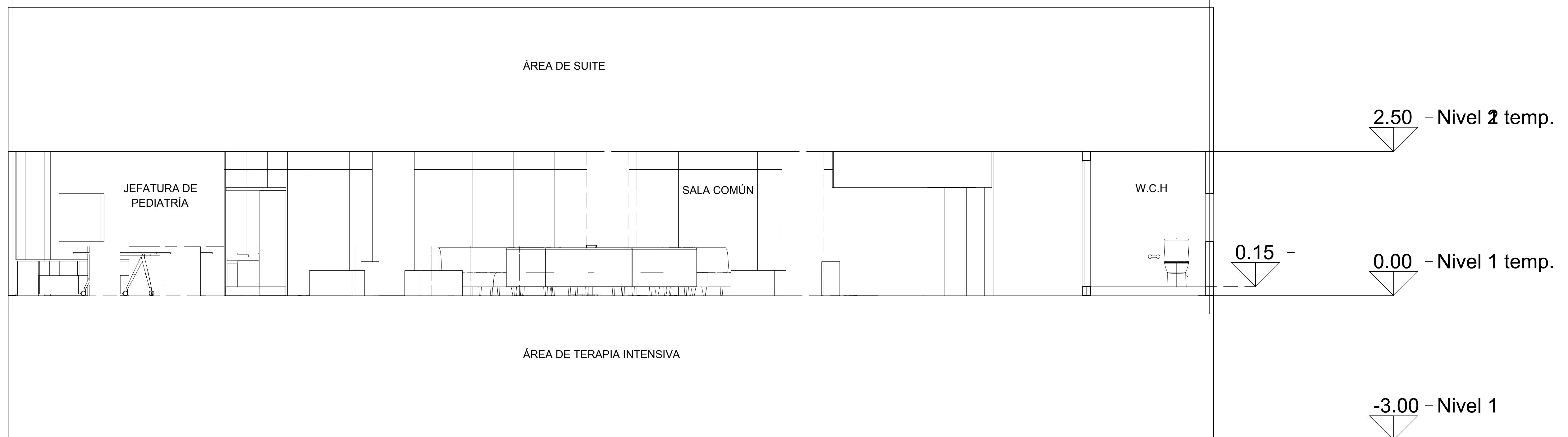
CORTE A-A' LONGITUDINAL
