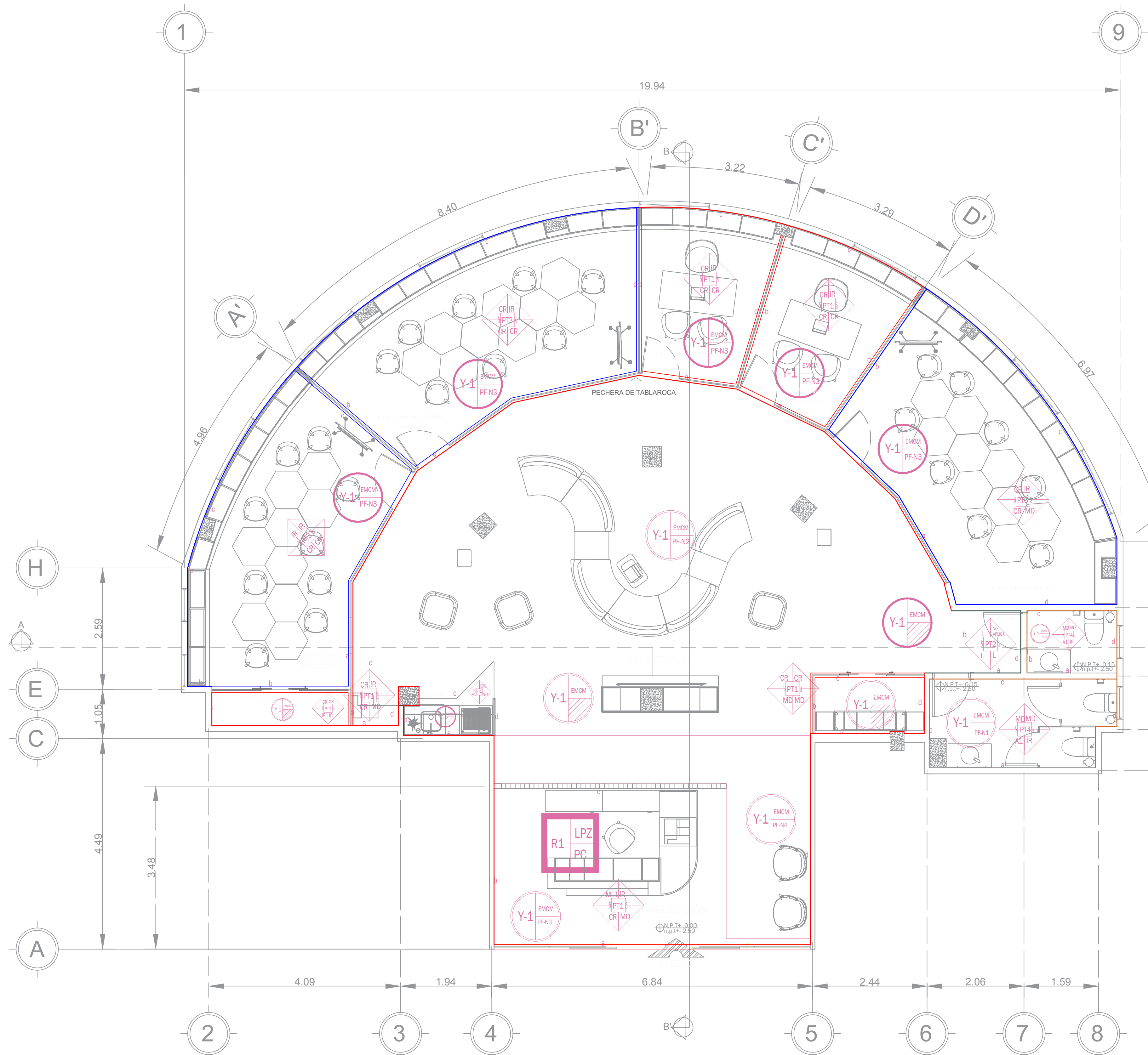
EDIFICIO HOSPITAL UNIVERSITARIO- ÁREA DE ENSEÑANZA E INVESTIGACIÓN
